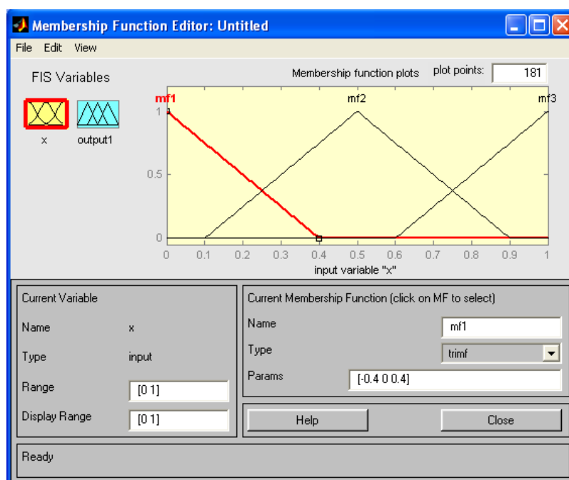
Рис. Окно редактора функций принадлежности
